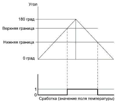
Рис.3. Принцип работы датчика в режиме контроля угла.
