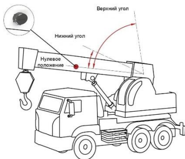
Рис.4. Размещение датчика DU-BLE в режиме угла.
