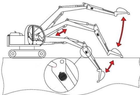
Рис. 5. Установка датчика DU-BLE на экскаватор
