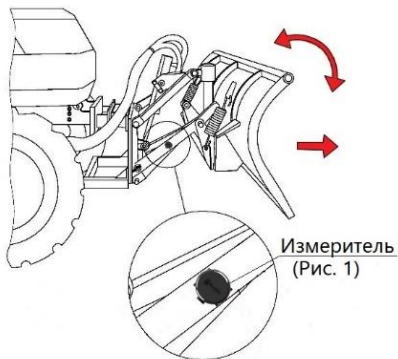
Рис.6. Установка датчика DU-BLE на устройства типа «отвал»
